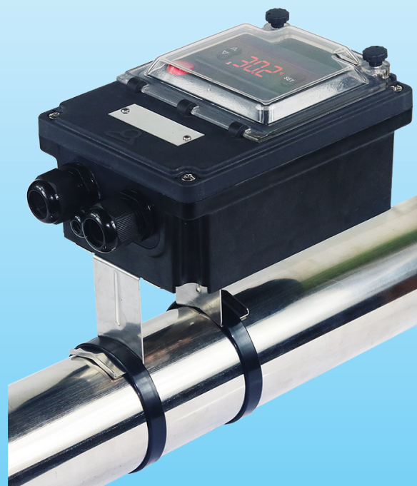
Esempio di montaggio con staffa posteriore su opzione tubo verticale
