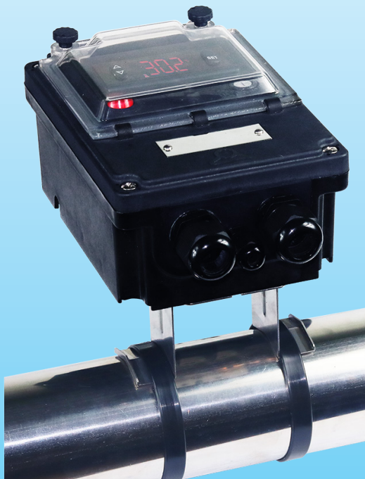
Esempio di montaggio con staffa di montaggio posteriore su opzione tubo orizzontale
